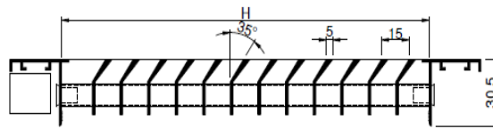
LM3 angle blade type
